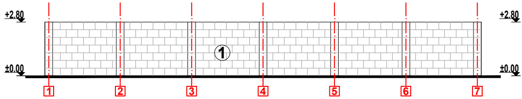
FATADA AX 1-7 - STATIE DE SORTARE SI INCINTE MATERIAL SORTAT
